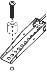
M8x25 (D)
